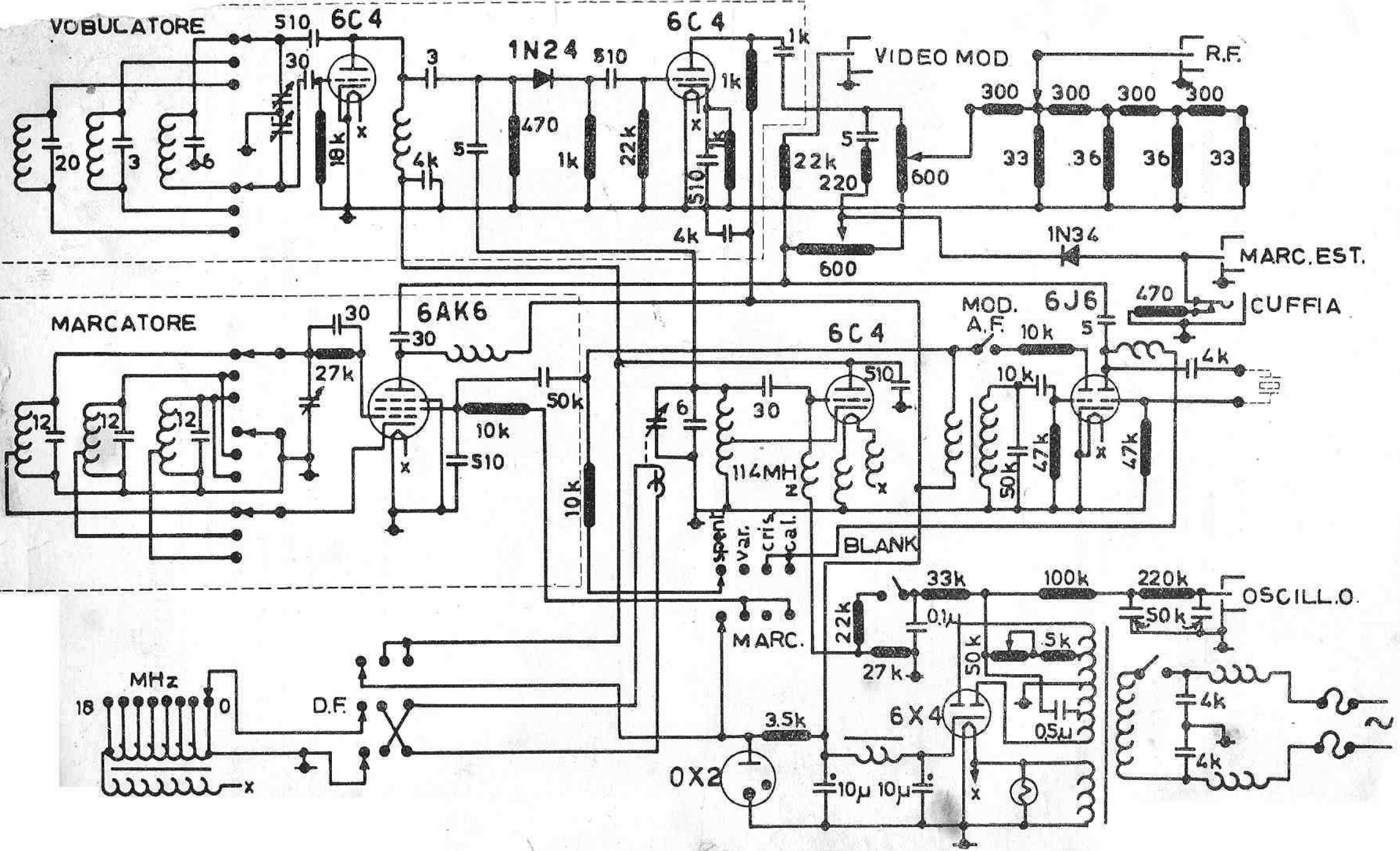
Fig. 78. - Vobulatore e marcatore Jackson TVG-2.
